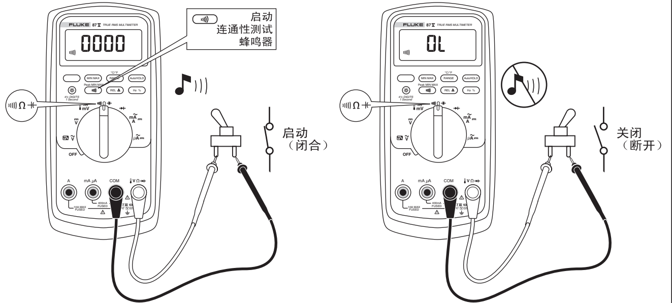
图4. 连通性测试
