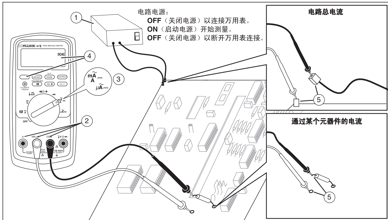
图8. 测量电流
