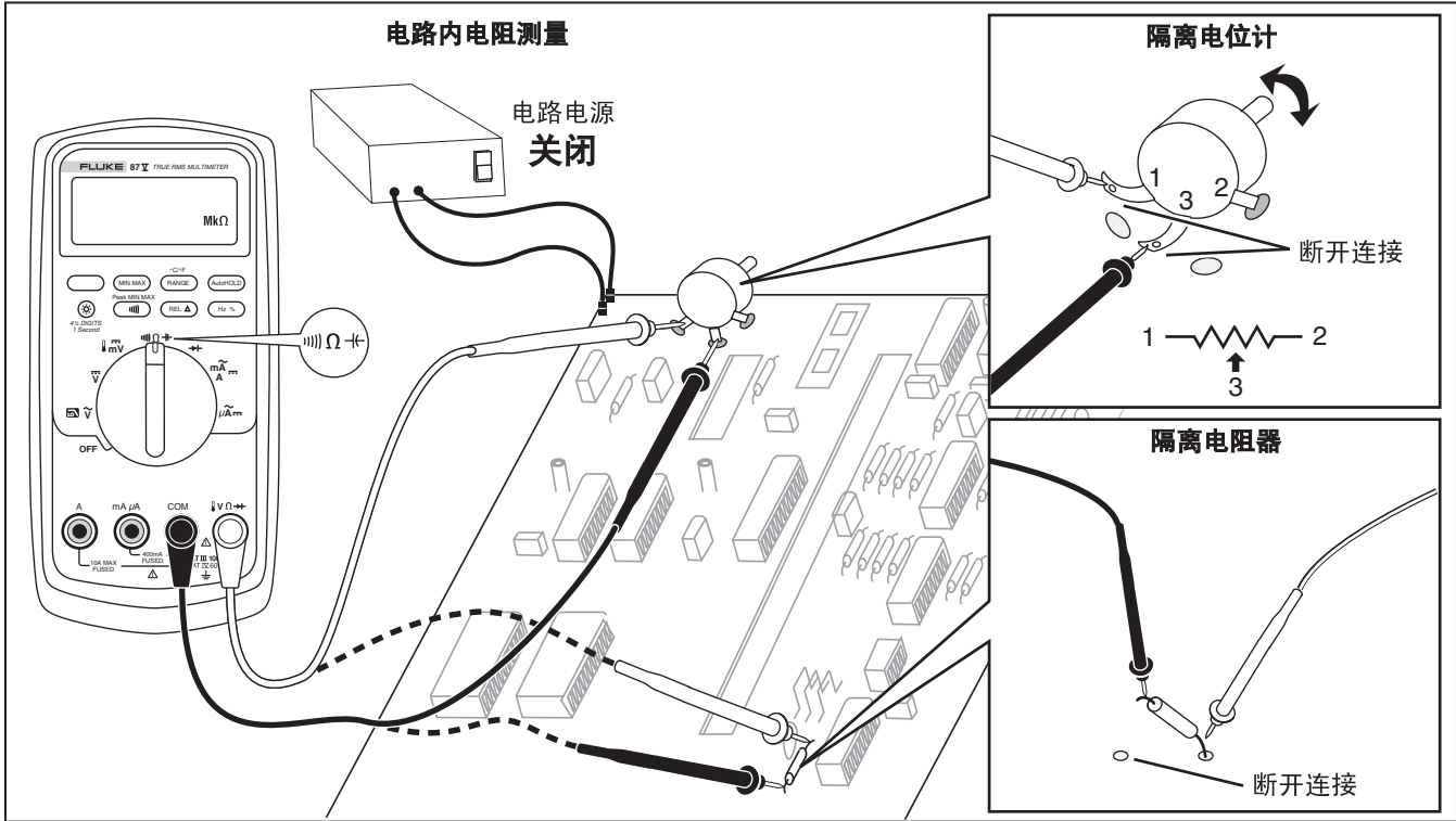
图5. 测量电阻
